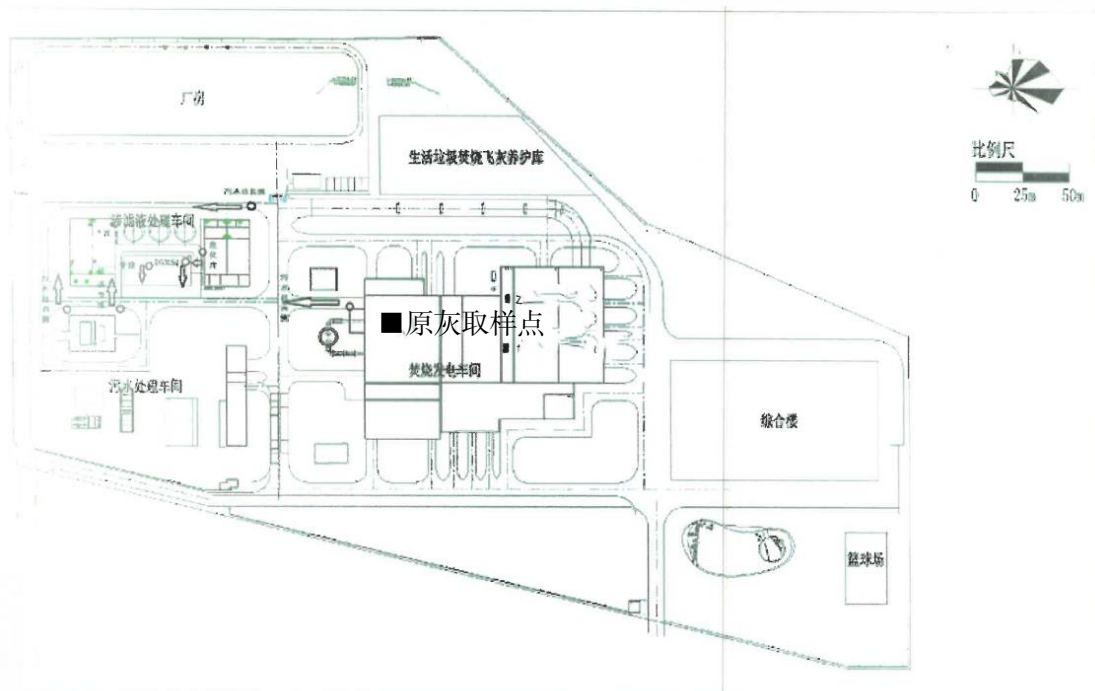
厂区平面图
