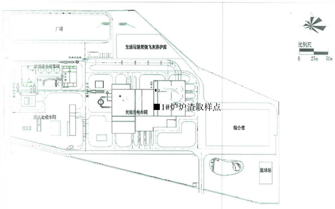
厂区平面图
